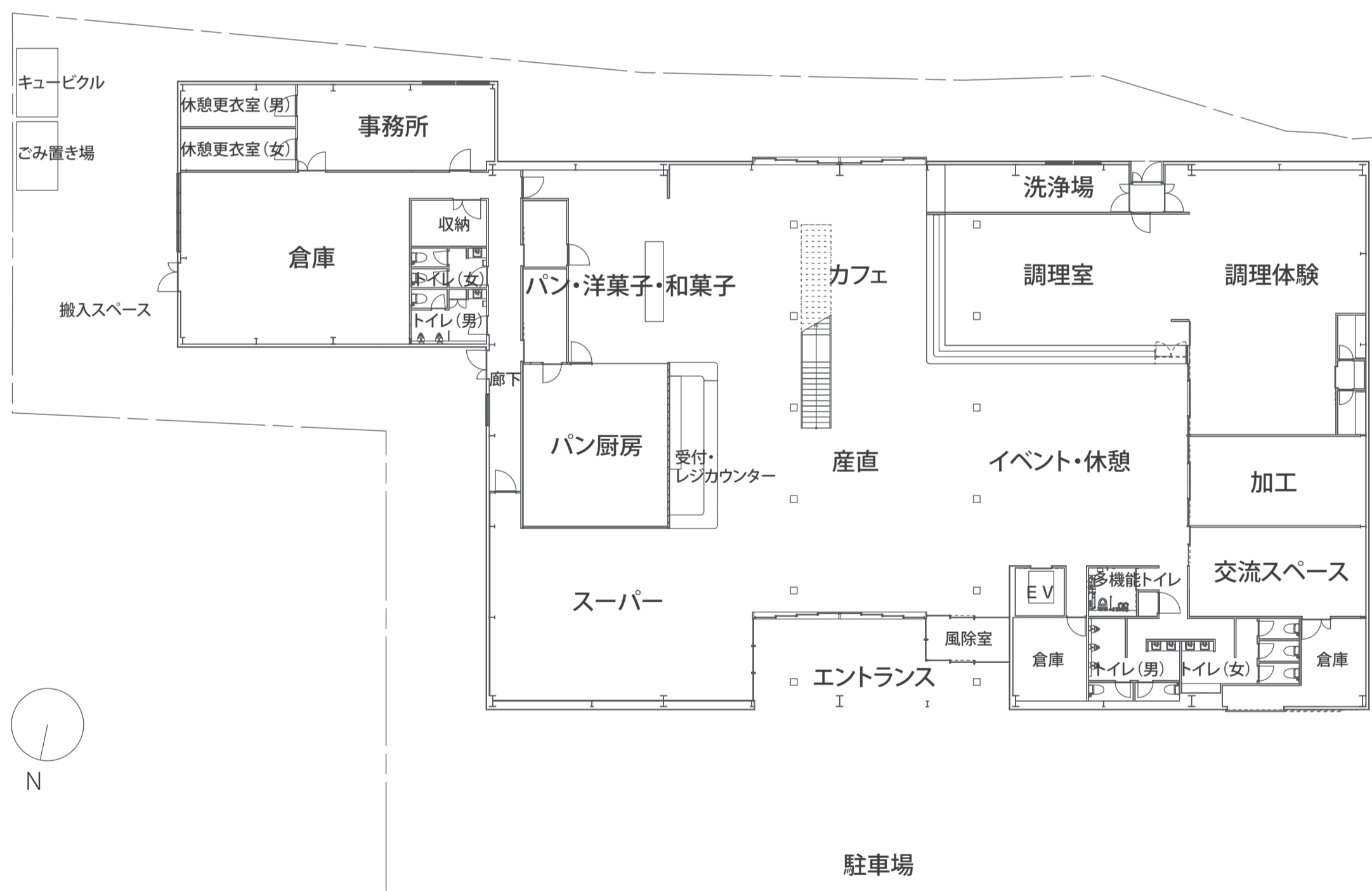
1F 平面図
